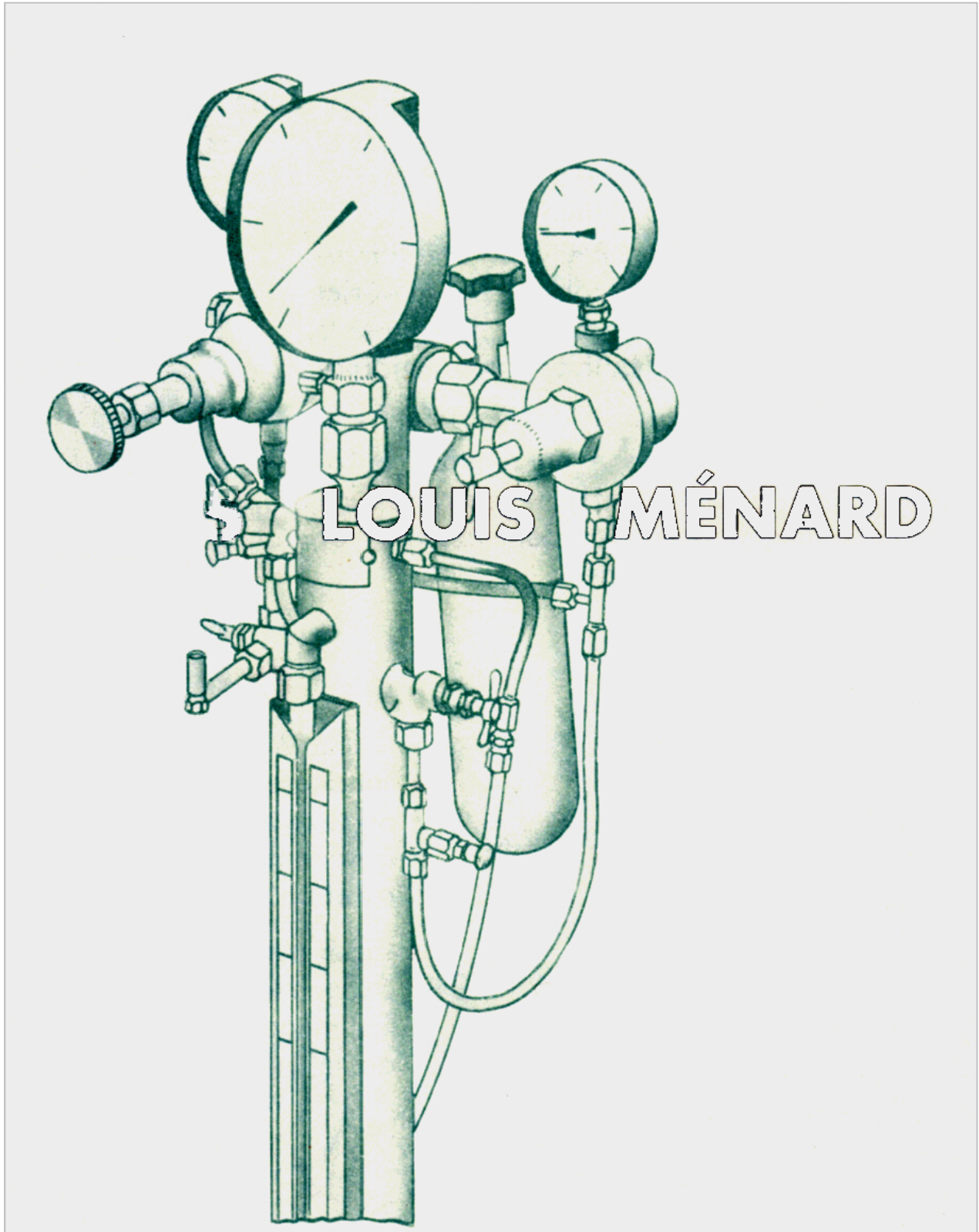
Le premier Pressiomètre ® type G. Modèle unique largement diffusé dès 1964, que les sondeurs avaient baptisé "le Mickey", à cause de ses deux oreilles. Les modèles carrossés apparaîtront dans les années 70. Dessin au crayon et fusain du bureau d'études Ménard, en couverture d'une brochure commerciale Études Pressiométriques Louis Ménard S.A.
