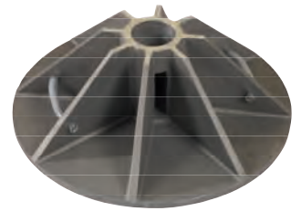
Plaque aluminium nervurée ø 600 mm
