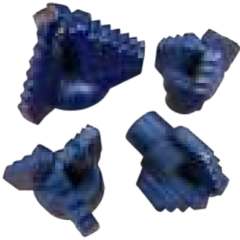
Trilames perdus avec carbures en divers diamètres
